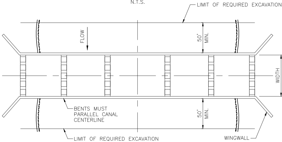
PLAN N.T.S.
