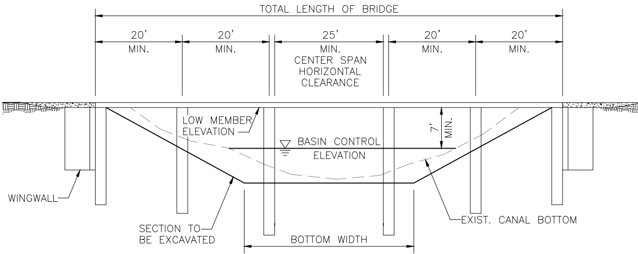
SECTION N.T.S.
