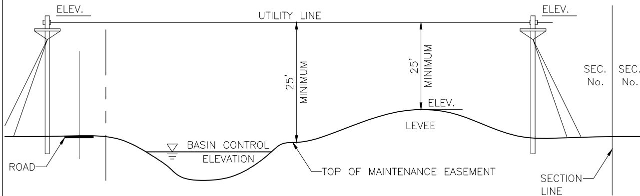
ELEVATION N.T.S.
